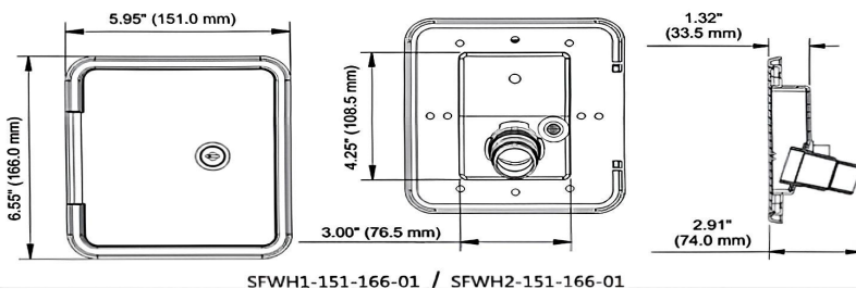
SFWH1-151-166-01 / SFWH2-151-166-01
