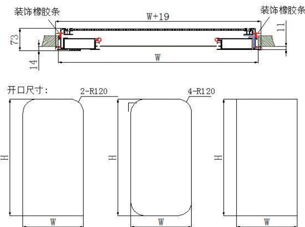
门吸（可选项）
